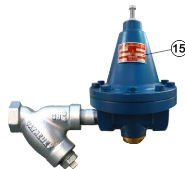
CONSTRUCCIÓN CON FILTRO TIPO "Y"
