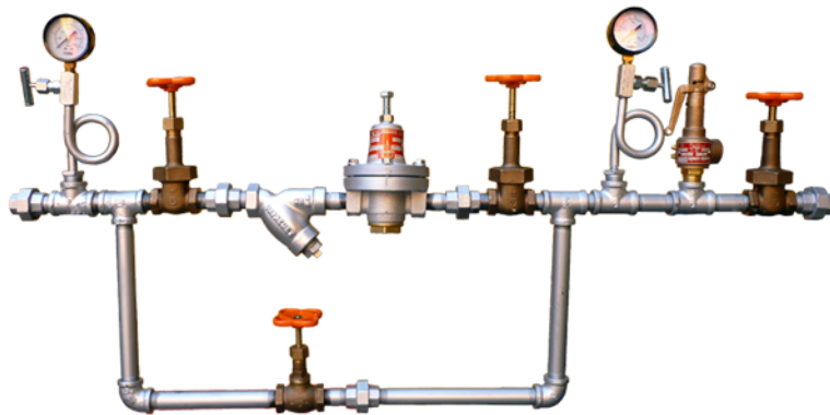
ESTACIÓN REGULADORA DE PRESIÓN MODELO ERP
